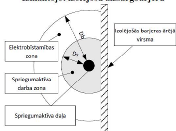
Sprieguma ietekmes zonu ierobežošana, Izmantojot izolējošu aizsargbarjeru
