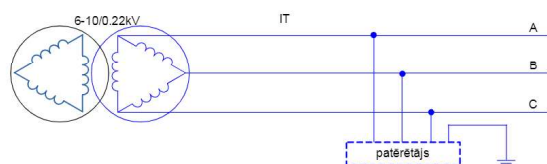
IT zemēšanas sistēma Rīgas pilsētas vēsturiskajā centrā
