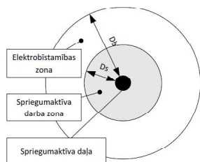
Attālumi gaisā un darba veikšanas zonas
