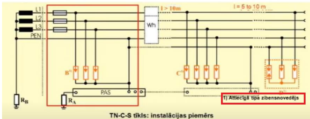
TN-C-S tīkls: instalācijas piemērs
